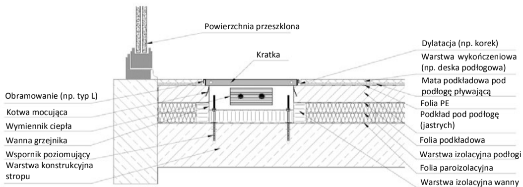
Przykład montażu grzejnika kanałowego VK15
